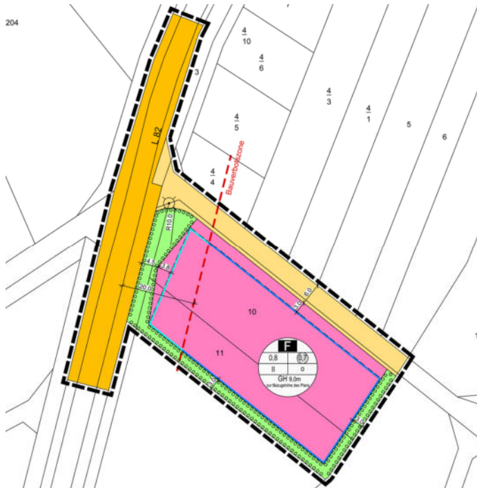
Abbildung 3: Entwurf der Planzeichnung für den BPL „Feuerwehrgerätehaus Waldorf“ (verändert nach Faßbender Weber Ingenieure PartGmbH).
